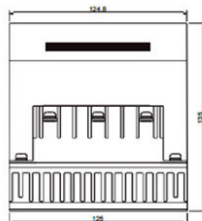
ESR30-75A Типоразмер C
