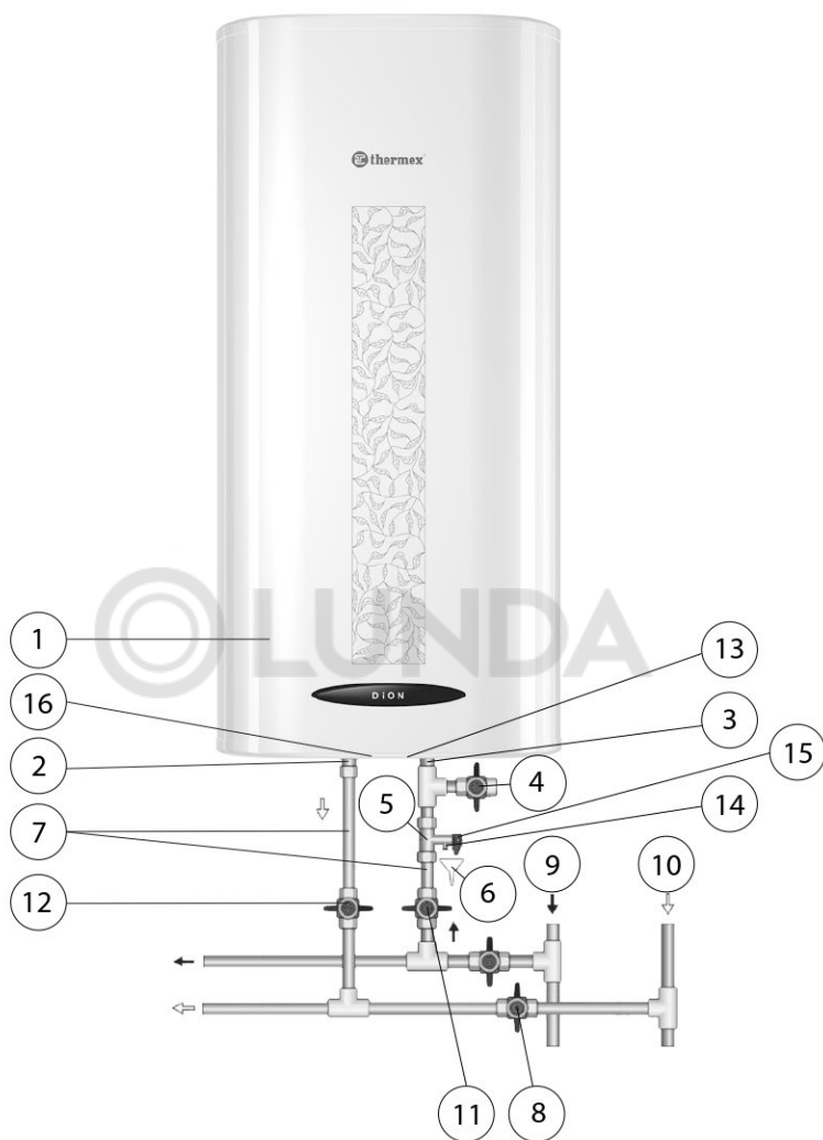
Рисунок 1. Схема подключения ЭВН к водопроводу в вертикальном положении
