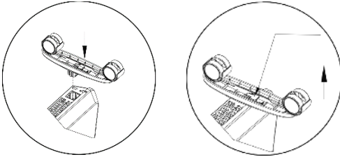
Рис. 1 Установка/снятие шасси
