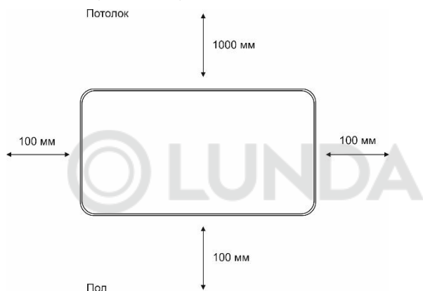
Рис. 3 Минимальное расстояние до посторонних предметов при настенной установке
