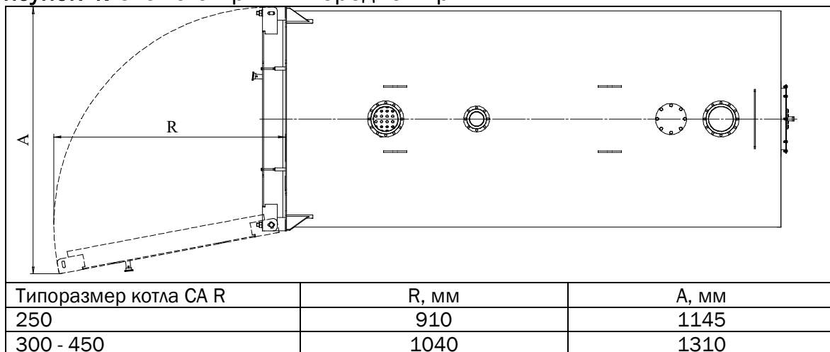
Рисунок 4. Схема открытия передней крышки
