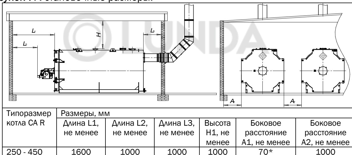
Рисунок 7. Установочные размеры.
