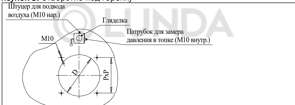
Рисунок 3. Отверстие под горелку
