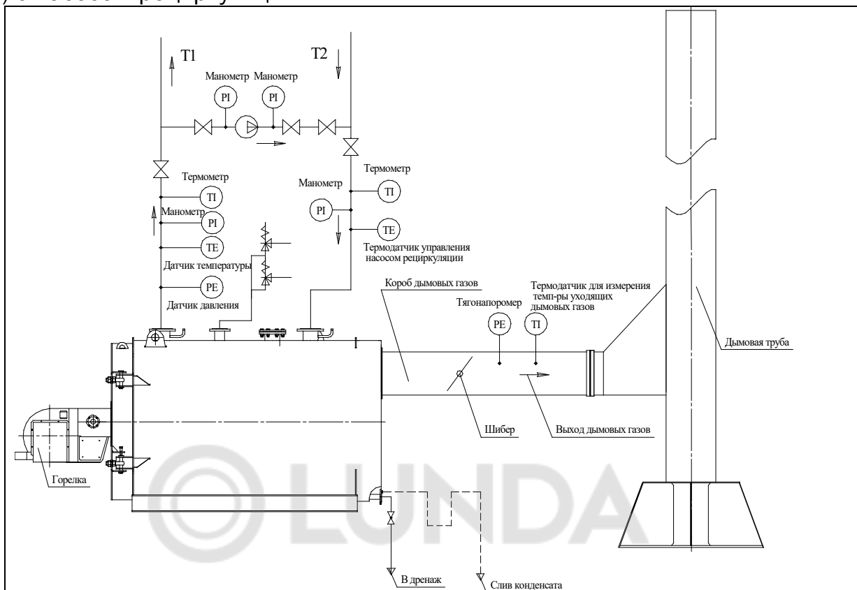
Рисунок 6. Принципиальные схемы включения котла
