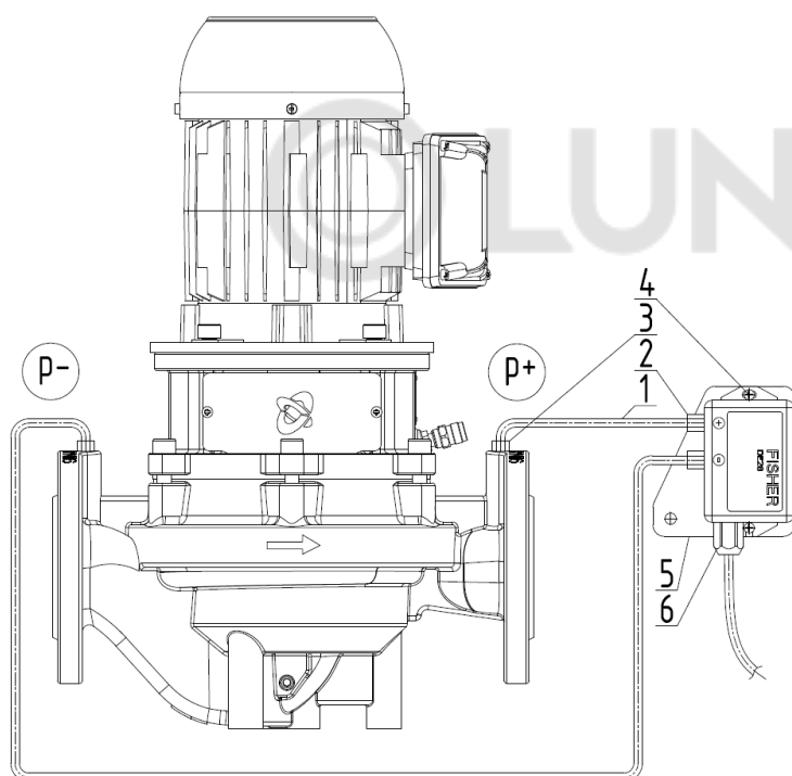
Abbildung 1: Schematische Darstellung der Montage des Druckmessers DE28
