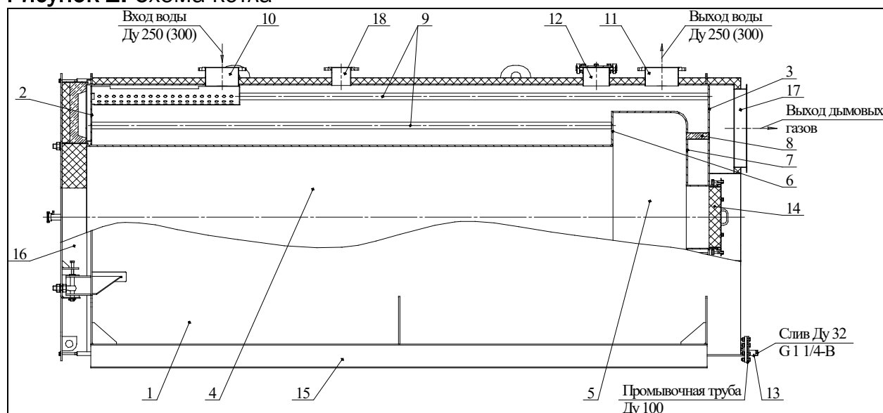
Рисунок 2. Схема котла
