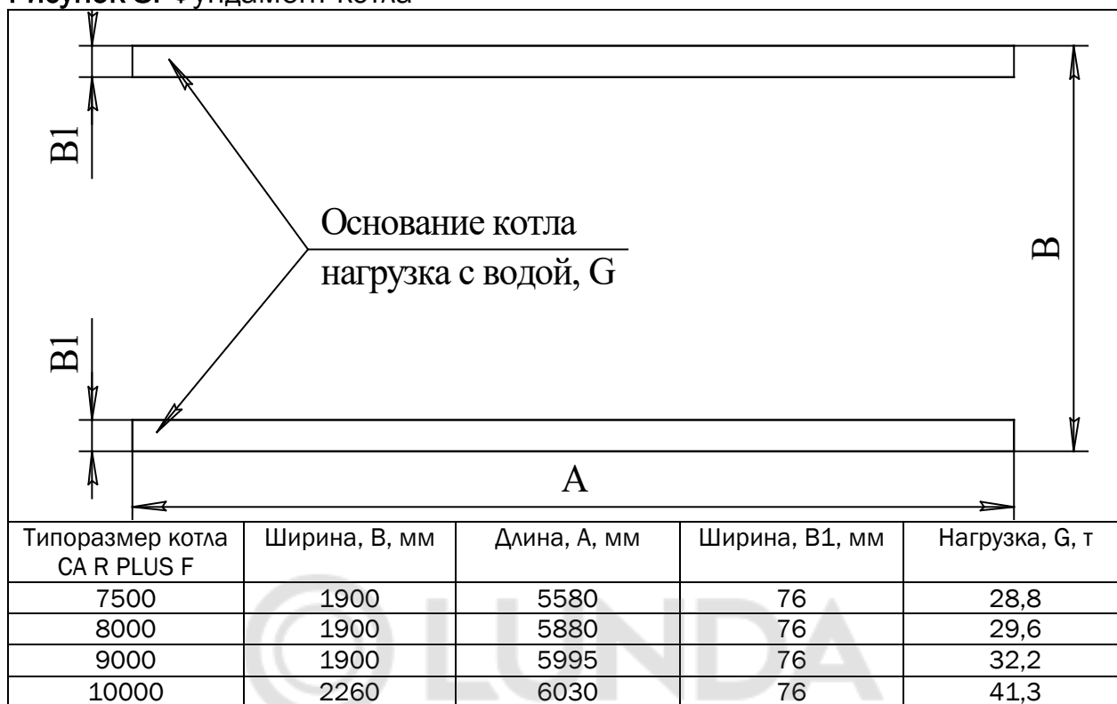
Рисунок 8. Фундамент котла
