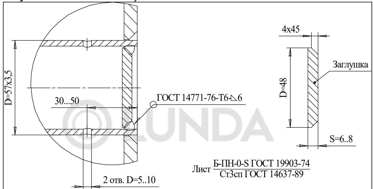
Рисунок 10. Установка заглушки
