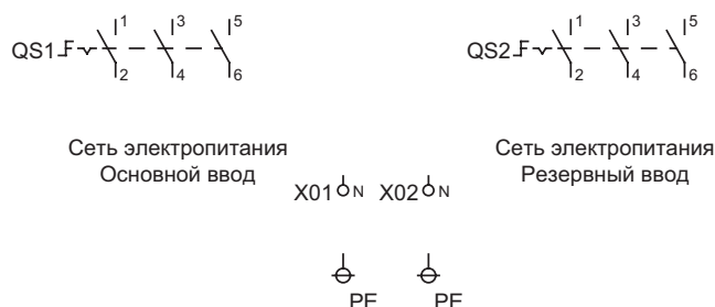
Рис. 36 Двойной ввод питания 3х380V, N, PE с АВР
