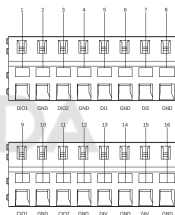
Рис. 44 Клеммы входов/выходов
