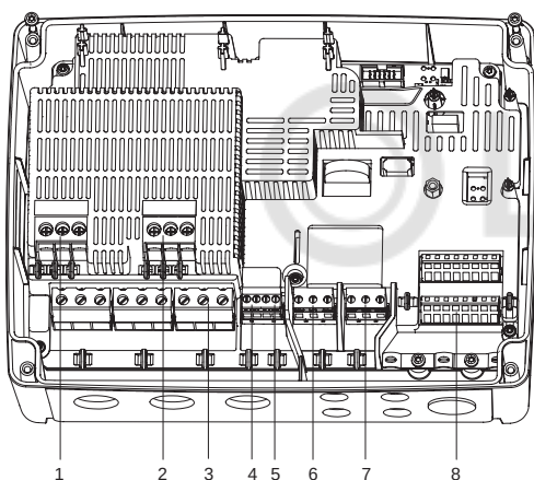
Рис. 42 Клеммные колодки
