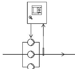
Рис. 5 Установка повышения давления
