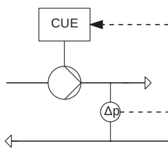
Рис. 89 Постоянный перепад давления, система
