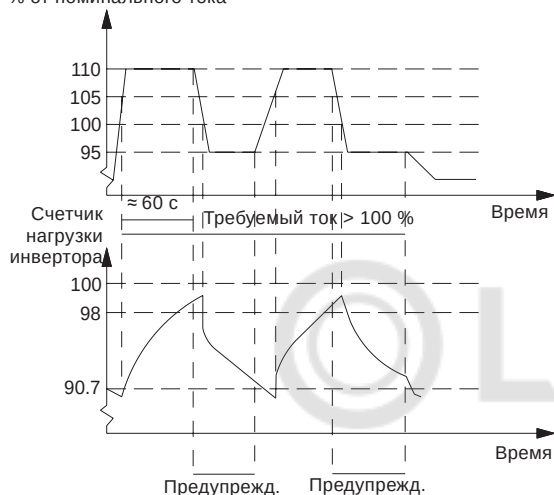
Рис. 114 Выходной ток в условиях перегрузки
