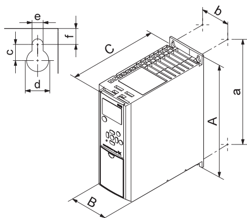
Рис. 136 Корпусы A2, A3 и B3
