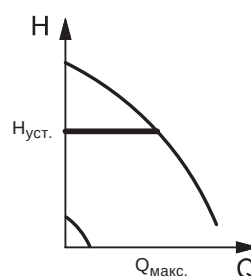
Рис. 88 Постоянный перепад давления, насос
