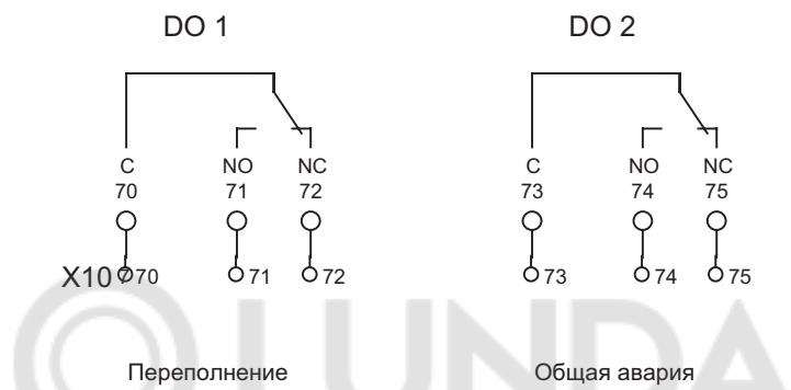
Рис. 67 Выводы сигнальных реле контроллера
