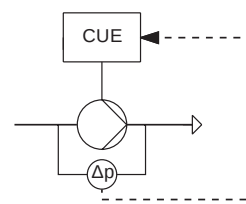
Рис. 88 Постоянный перепад давления, насос
