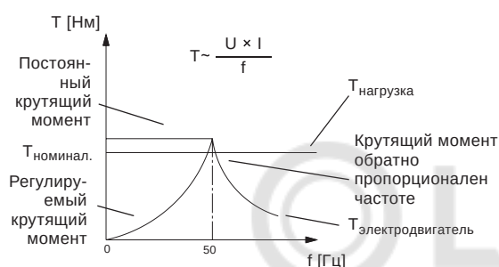
Рис. 113 Регулирование по характеристике T/n (идеальное)
