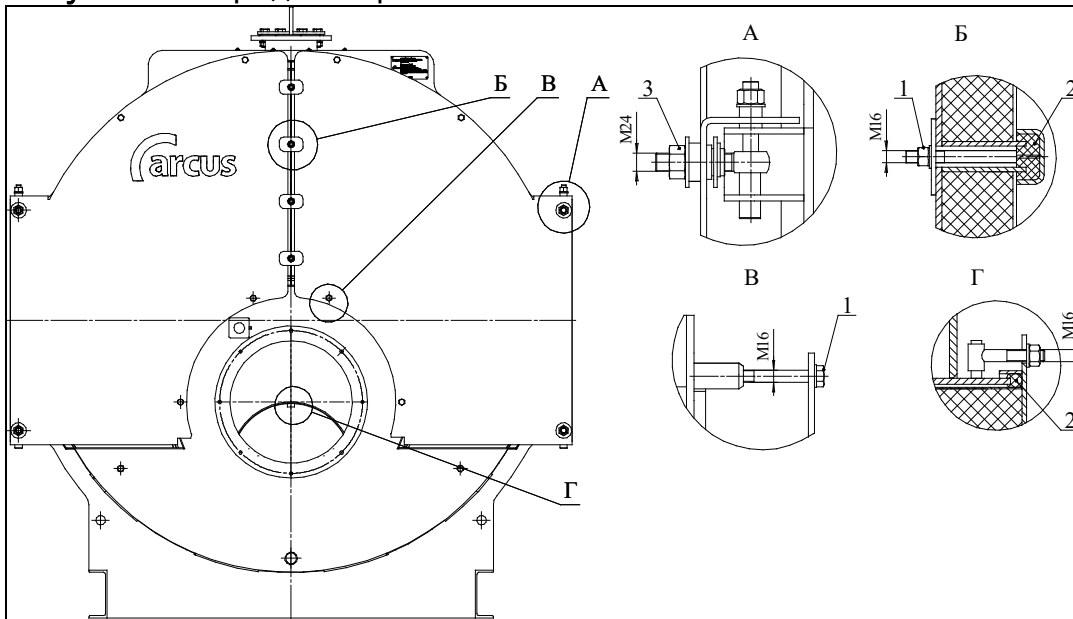
Рисунок 9. Передние крышки
