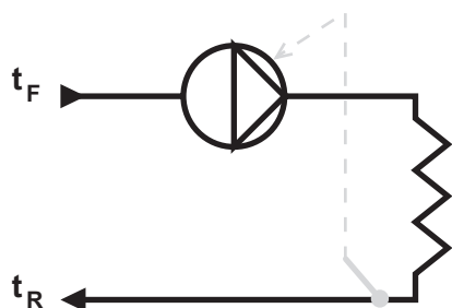
Рис. 53 Насос с внешним датчиком
