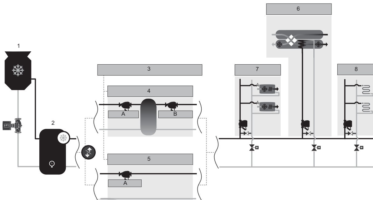
Рис. 46 Функциональная схема системы охлаждения в коммерческом здании
