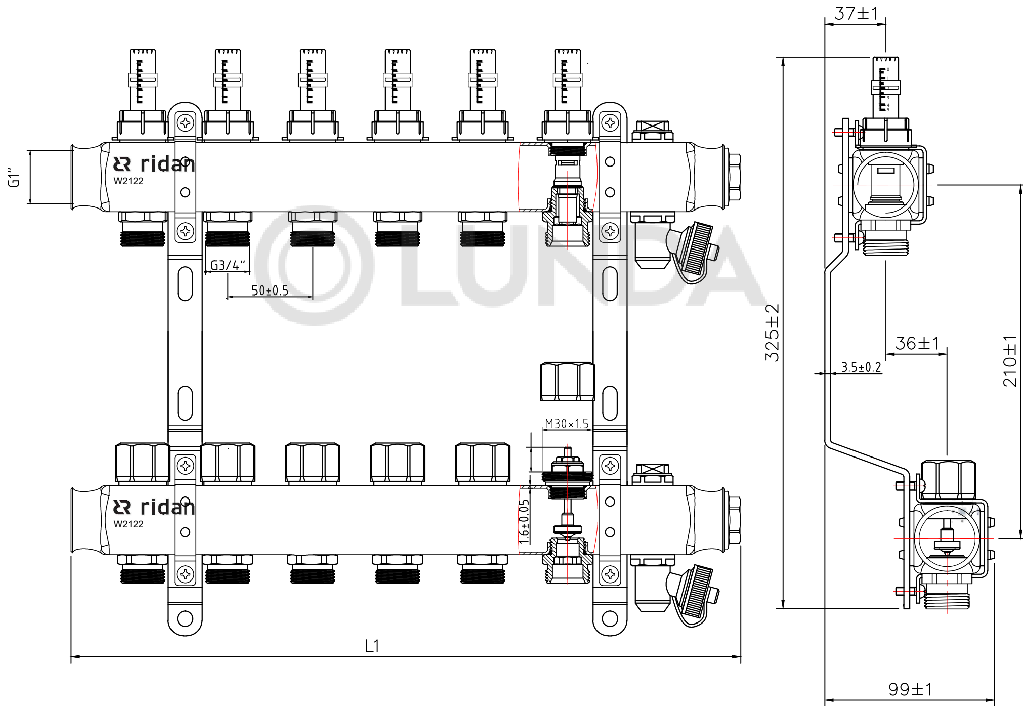
Габаритные размеры
