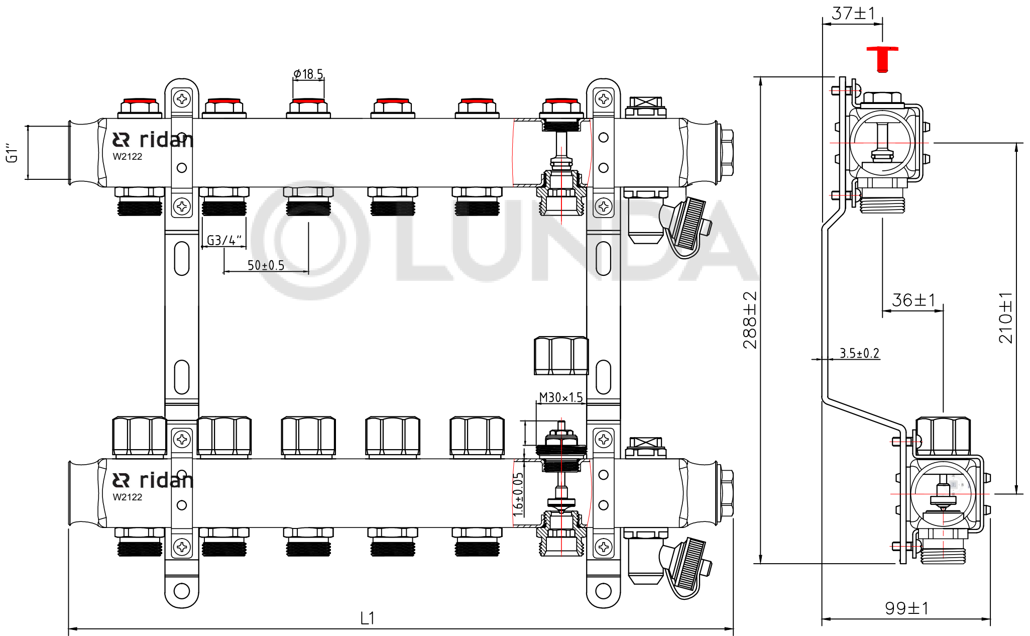
Габаритные размеры
