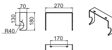
Кронштейн для гидроразделителя универсального, до 300 кВт
