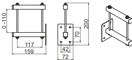
Кронштейн универсальный
