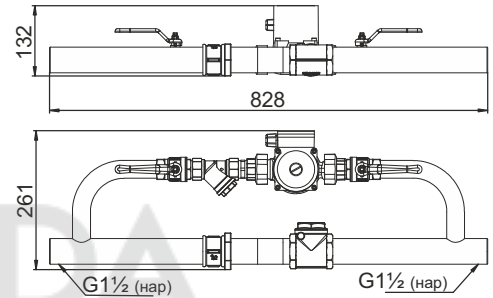
Насосный узел горизонтальный 25-60/40
