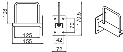
Кронштейн со скобой настенный универсальный
