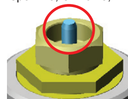
Выемка для захвата и вытягивания штифта клапана
