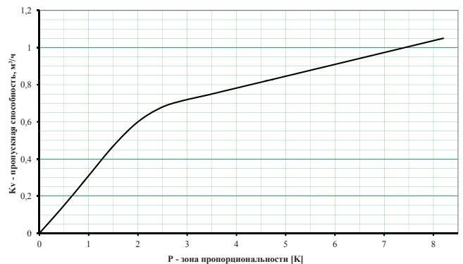
Область пропорционального отклонения - это технико-регулируемый показатель температурного отклонения (K), когда радиаторный терморегулятор приводится в действие термостатической головкой. В соответствии с располагаемым на клапане перепадом давления задаётся пропорциональное отклонение. Для подбора радиаторных терморегуляторов рекомендуется область пропорционального отклонения от 0,5 К до 2 К.
