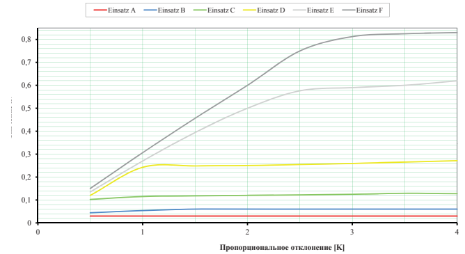
Клапаны, отличающиеся большим конусом, особенно удачно подходят для систем с малым расходом, т.к. при малых значениях преднастройки нет необходимости принимать во внимание технологические допуски.
