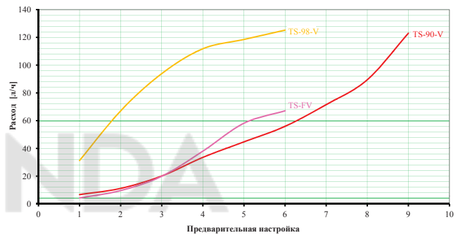
Клапаны с преднастройкой, даже при равной номинальной максимальной пропускной способности, чётко отличаются по градиции преднастройки для того, чтобы соответствовать различным требованиям и целям применения.
