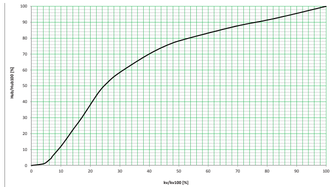
Характеристика клапана показывает зависимость степени открытия от расхода. Показанная линия типична для радиаторных терморегуляторов с малым ходом штока.
