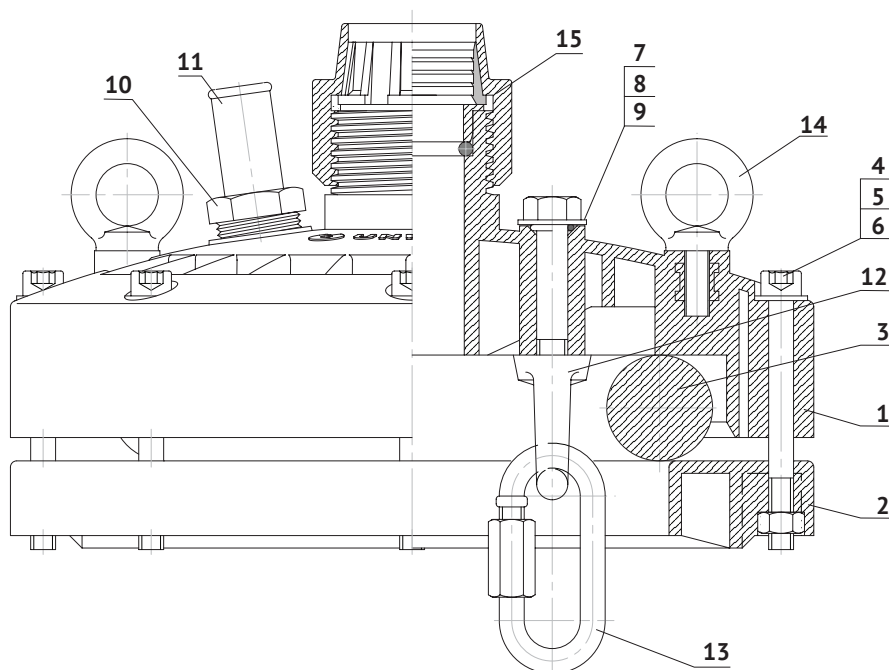
Рисунок 1 - Устройство оголовка
