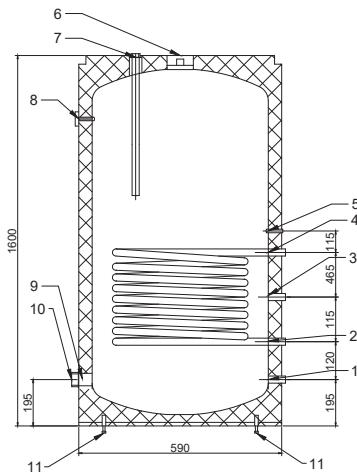
Рис. 3. Размеры SWH-2110-300
