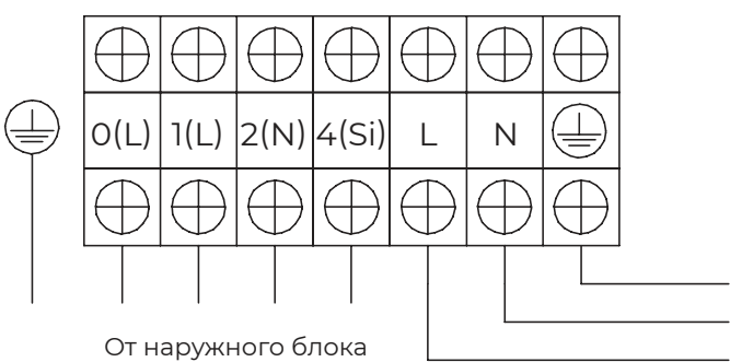
Клеммный терминал наружного блока
