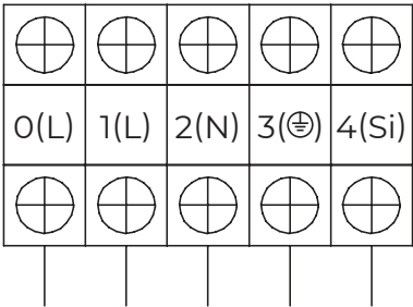
Клеммный терминал внутреннего блока
