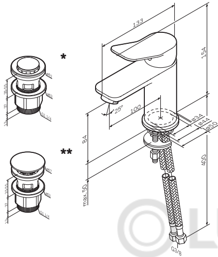
X-Joy F85A021XX F85A028XX F85A82100*/XX** F85A82800*/XX**
