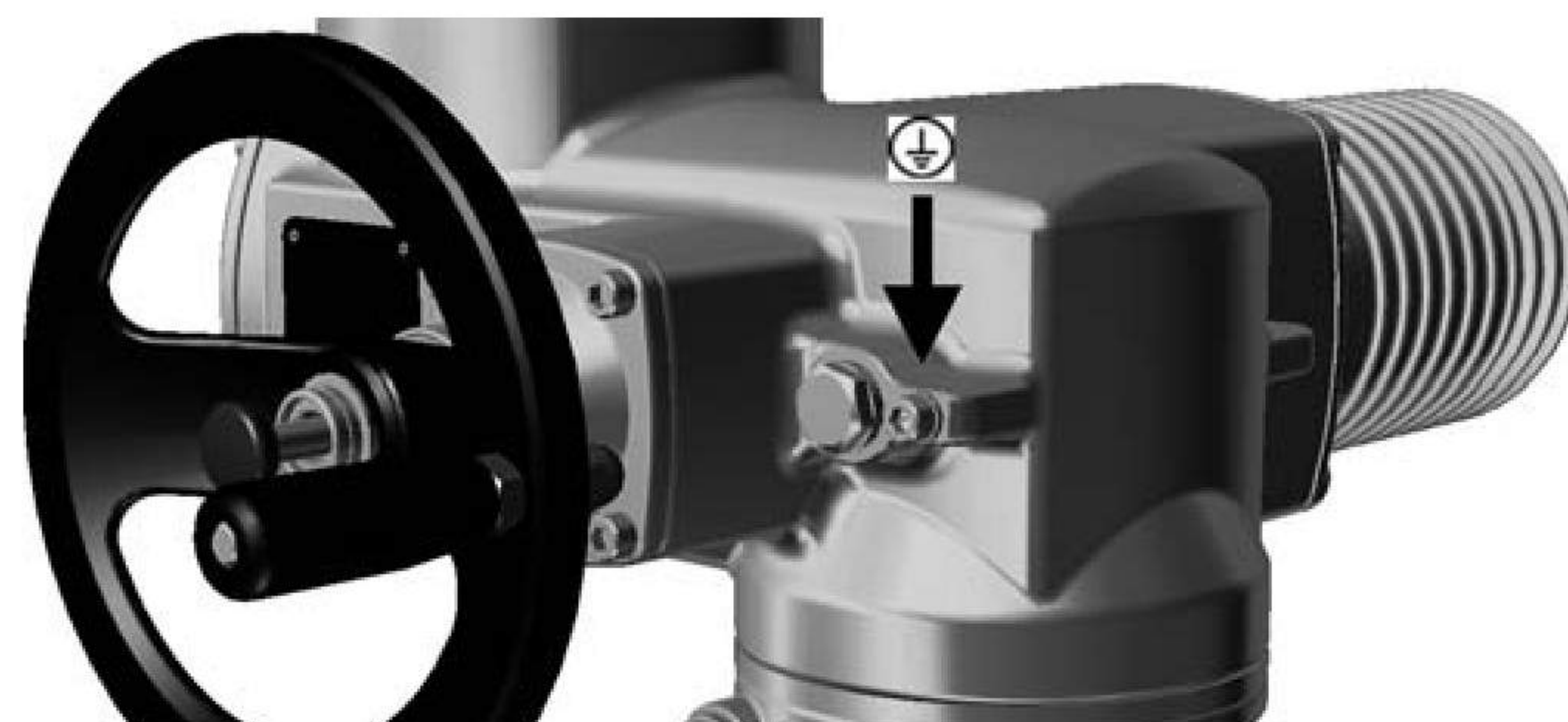
рис. 13: Контакт заземления
