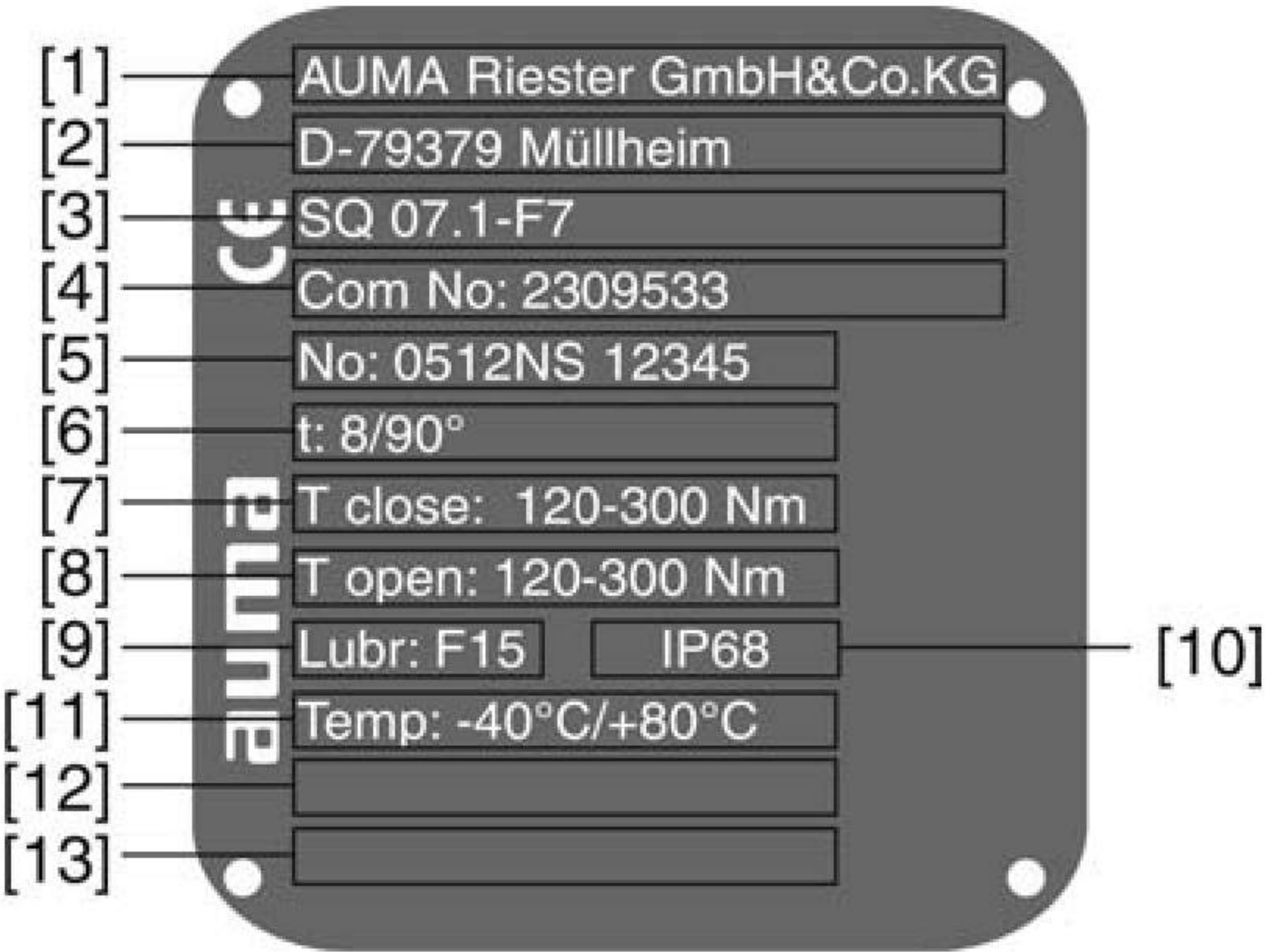
рис. 2: Заводская табличка привода (пример)
