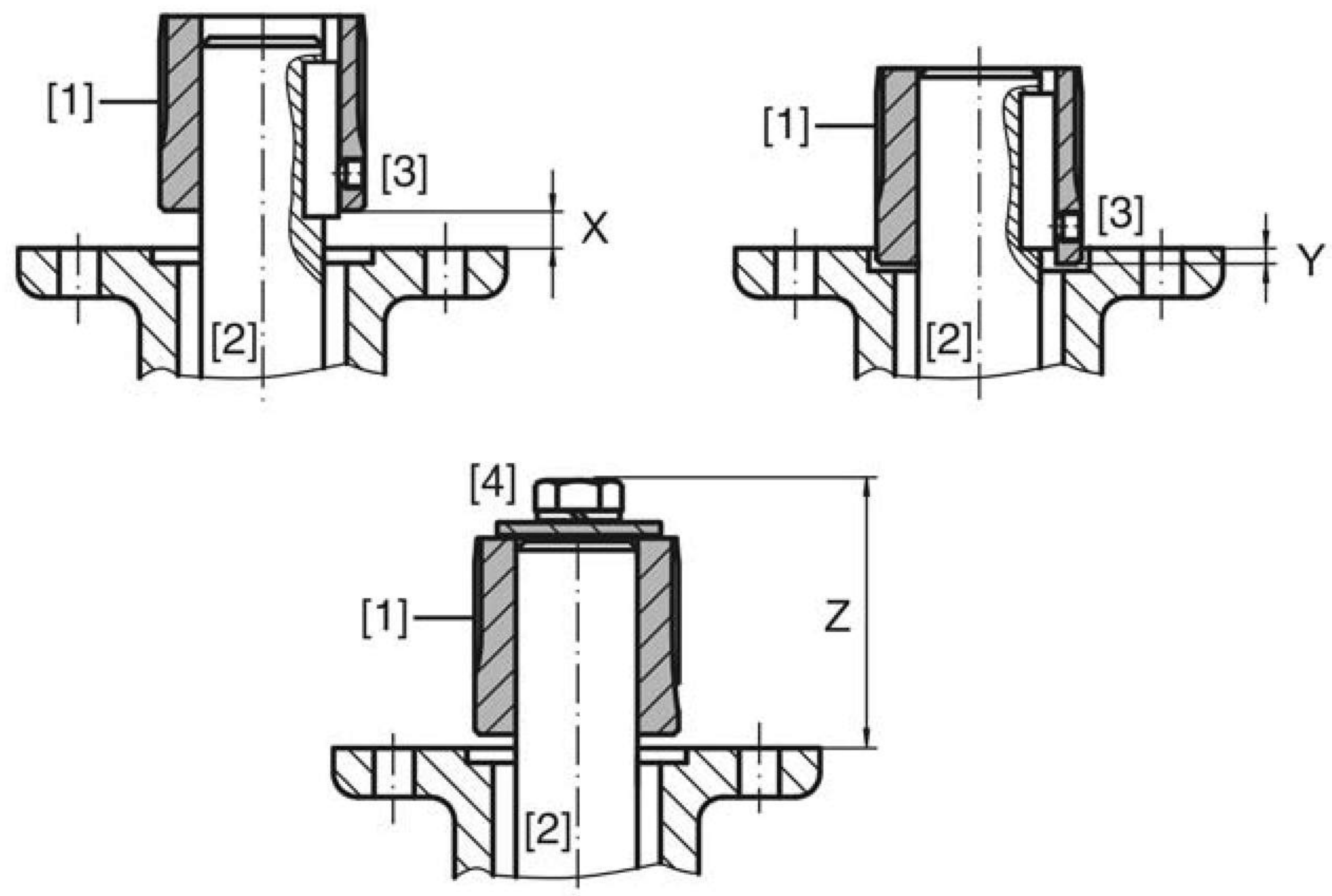
рис. 5: Установочные размеры втулки
