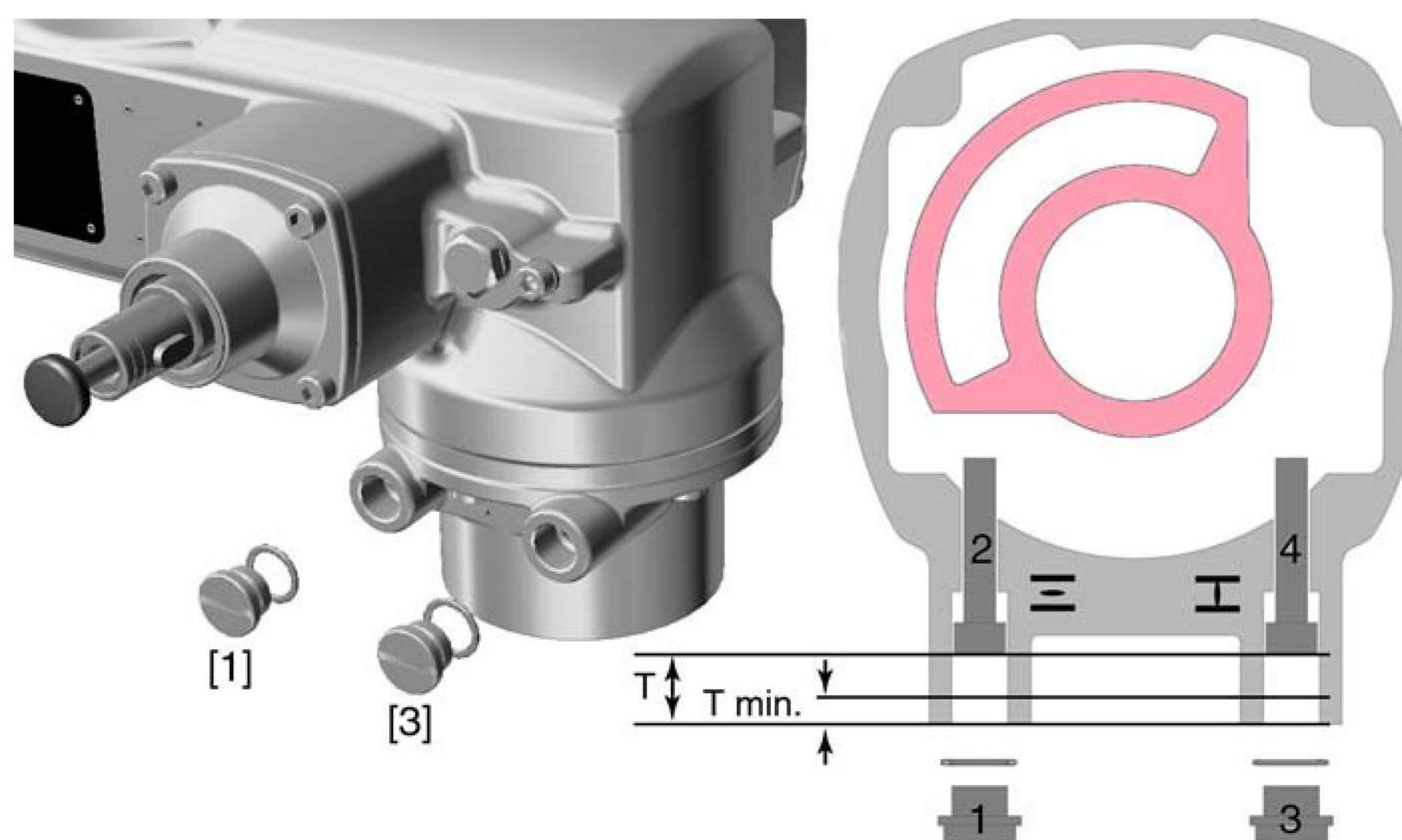
рис. 17: Концевой упор
