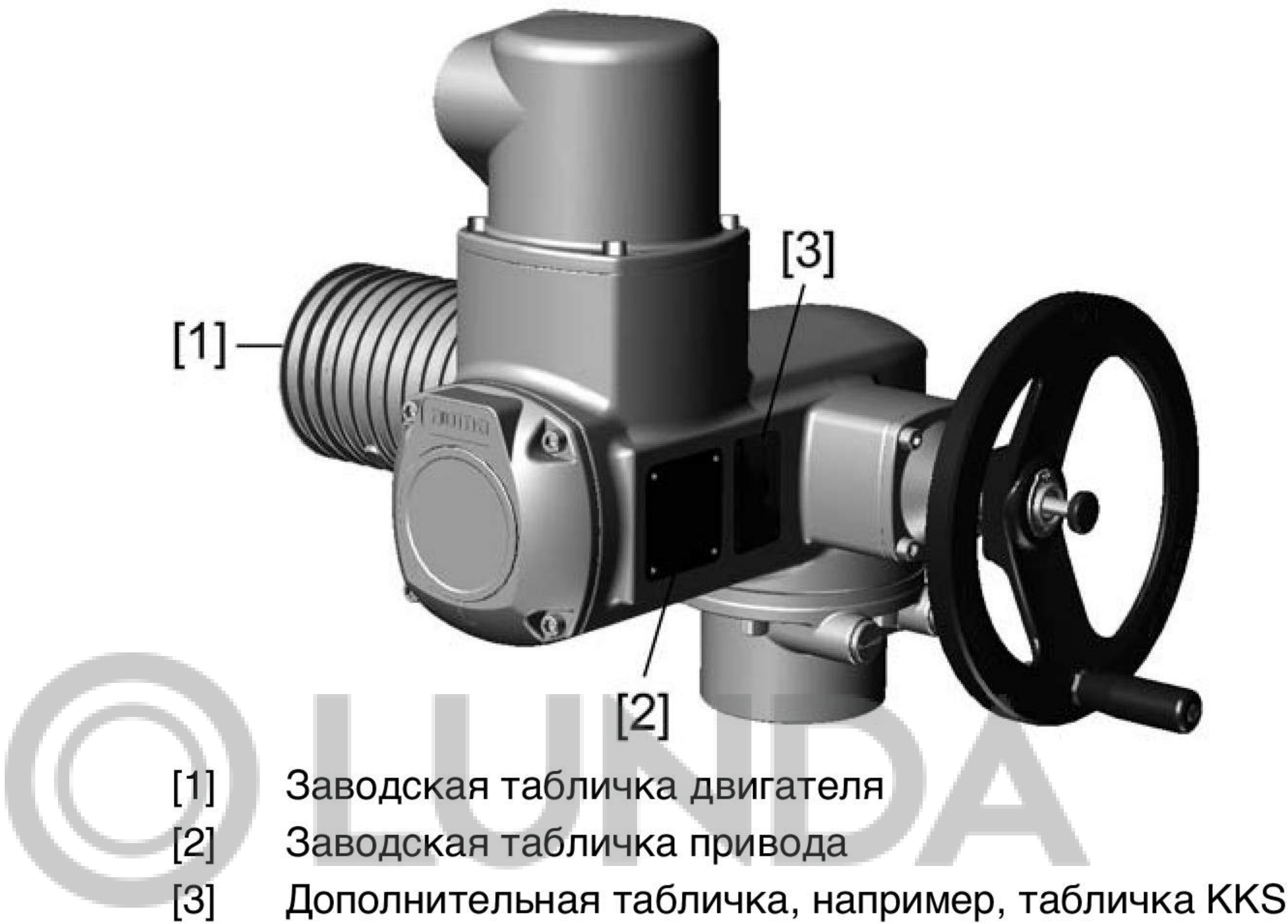
рис. 1: Вид заводской таблички
