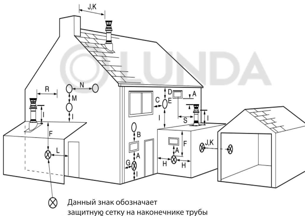
Рисунок 4. Рекомендуемые отступы дымохода.
