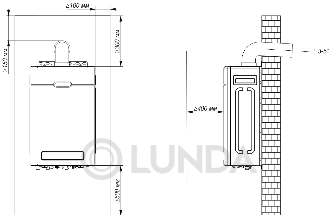
Рисунок 3. Пространство для технического обслуживания.
