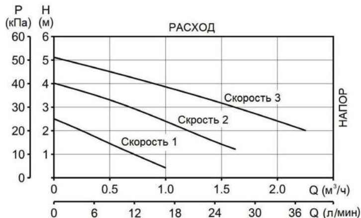
Рис. 18 Напорно-расходные кривые циркуляционного насоса электродкотла.
