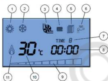
Рис. 6 ЖК-дисплей панели управления электродкотлом
