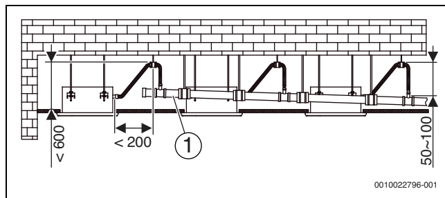
Рис. 30 Расстояние до сливного трубопровода (мм)
