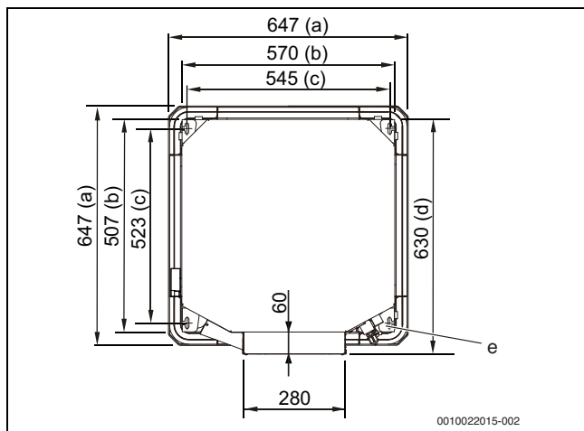
Рис. 14 Размеры блока (мм)
