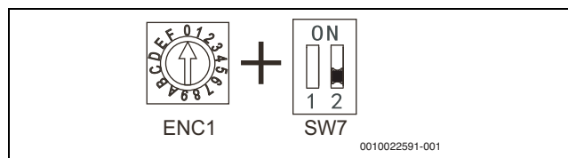
Рис. 42 ENC1 + SW7_2
