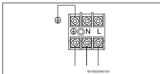
Рис. 35 Входное питание
