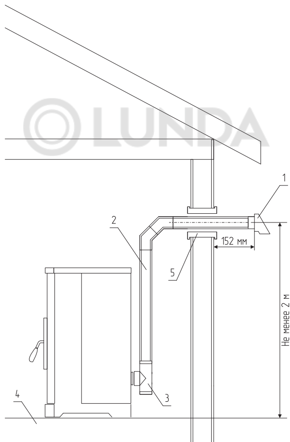
Рис.8 Подключение дымохода через стену
