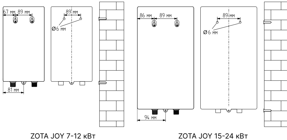
Рис.4 Порядок установки: шаг 1
