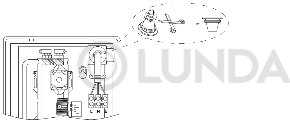
Рис.8 Обрезка резиновой водонепроницаемой втулки
