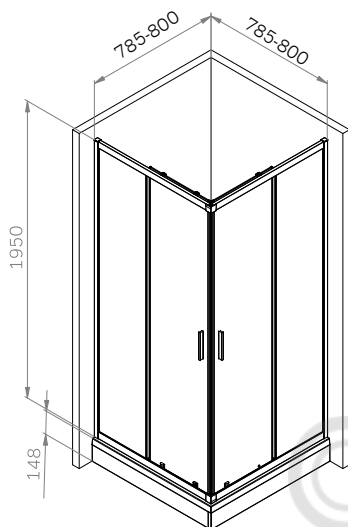
W90G-403-8080-MT W90G-403-8080-BT
