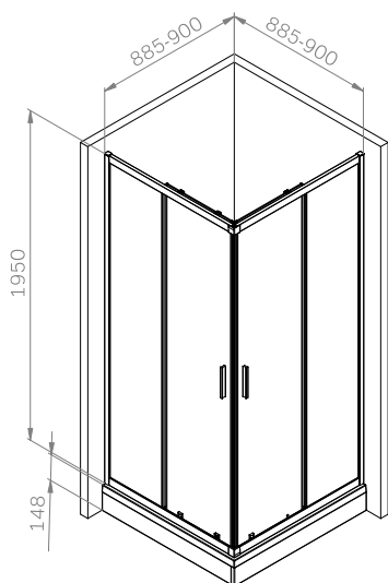
W90G-403-9090-MT W90G-403-9090-BT
