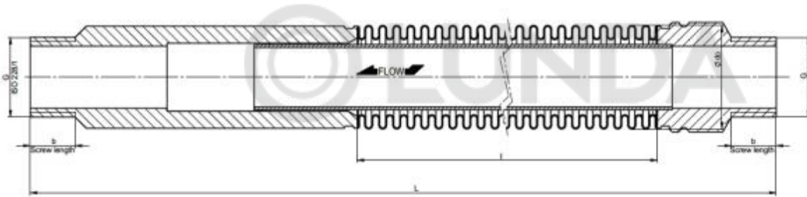
Осевой компенсатор с внутренней гильзой и без защитного кожуха.
