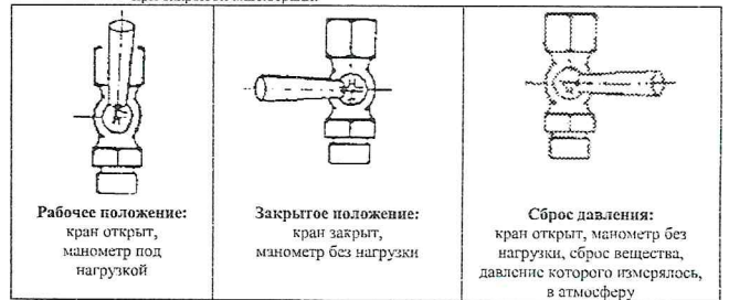
Рабочее положение: кран открыт, манометр под нагрузкой
