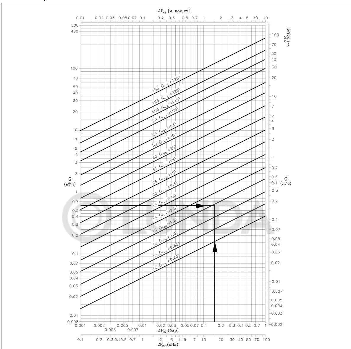
Рис. 6. Выбор типоразмера клапана.
