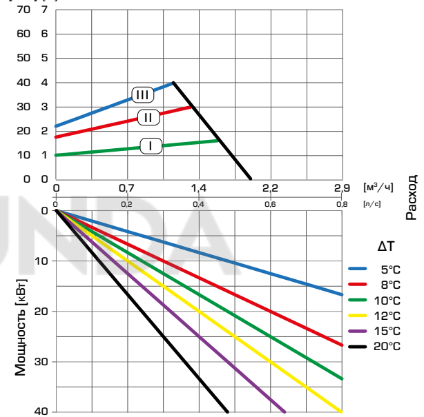
СЕРИЯ GFA394 — переменный перепад давления, насос Wilo ДР Напор [кПа] [м]
