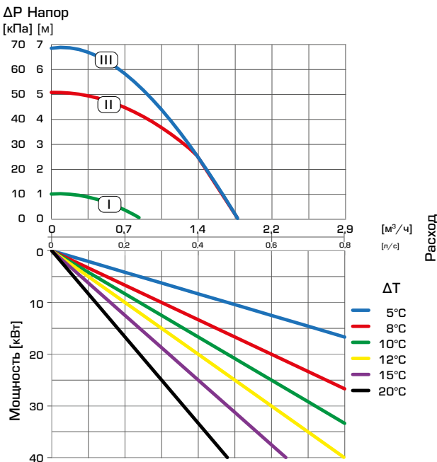
СЕРИЯ GFA394 — фиксированная скорость, насос Wilo ДР Напор [кПа] [м]
