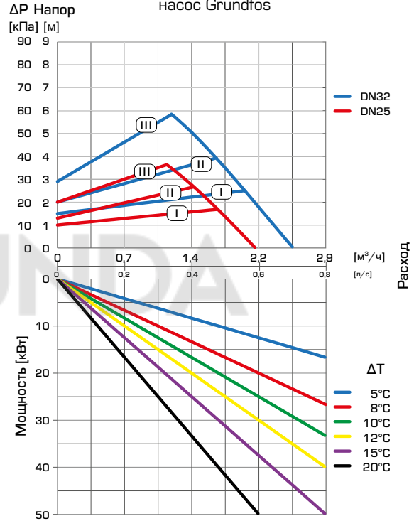
СЕРИЯ GFA212 — переменный перепад давления, насос Grundfos
