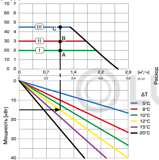
СЕРИЯ GFA394 — постоянный перепад давления, насос Wilo ДР Напор [кПа] [м]
